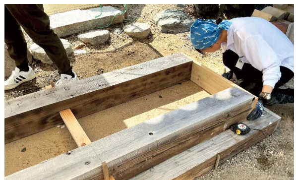
版築の型枠
